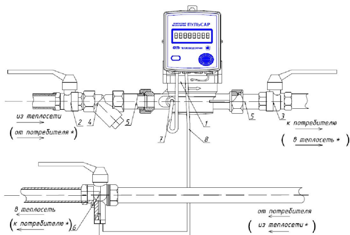
1-Теплосчётчик; 2,3-Кран шаровый; 4- Фильтр; 5-Комплект присоединительный; 6-Кран шаровый с отводом для термометра; 7,8-Термометр сопротивления
